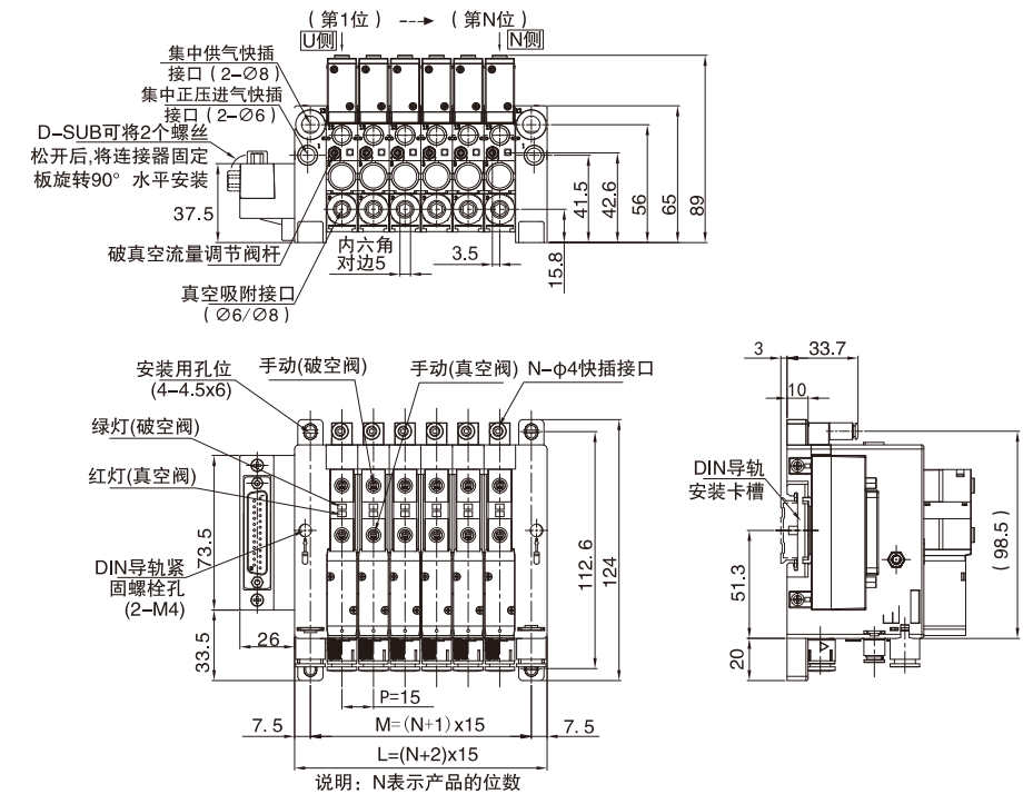
EZPV□-W 帶外接真空检测外形图
