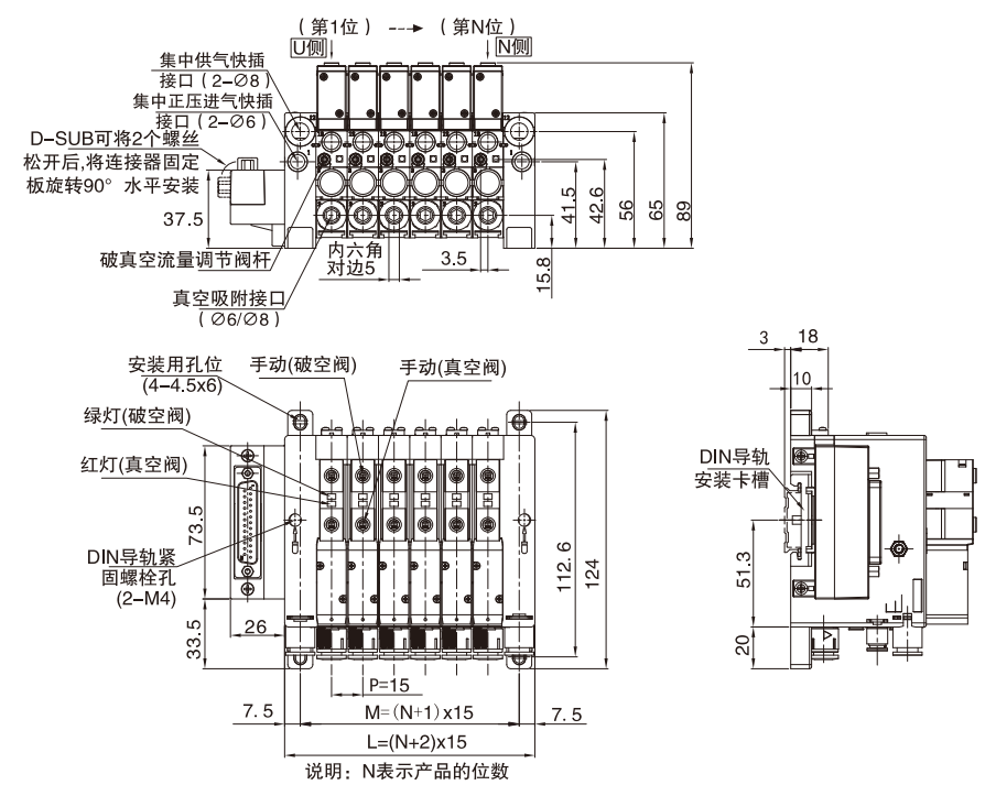
EZPV□ 不帶真空压力表外形图
